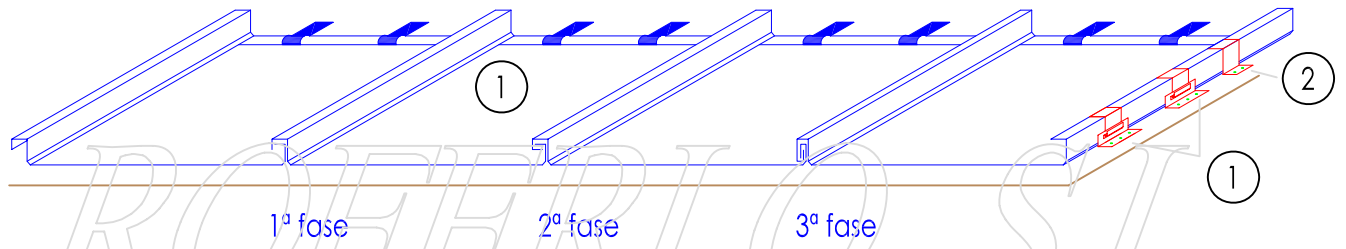
Sistema de Colocación de Bandejas y Fases de Engatillado
